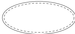
楕円形38.8×16.5mm (ゴルフマーカークリップ部)
